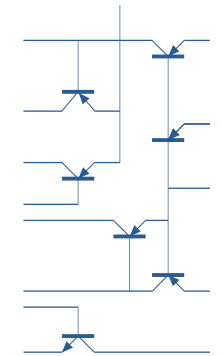
S12 (1 x NPN + 6 x PNP)
