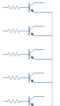
S8 (5 x NPN)
